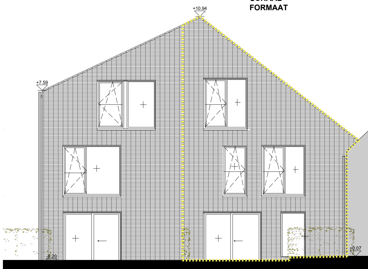
ZUID GEVEL
