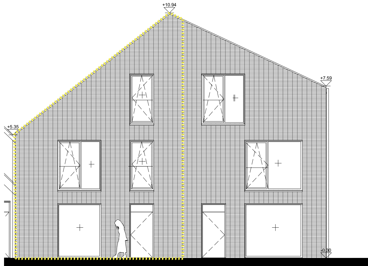
NOORD GEVEL
