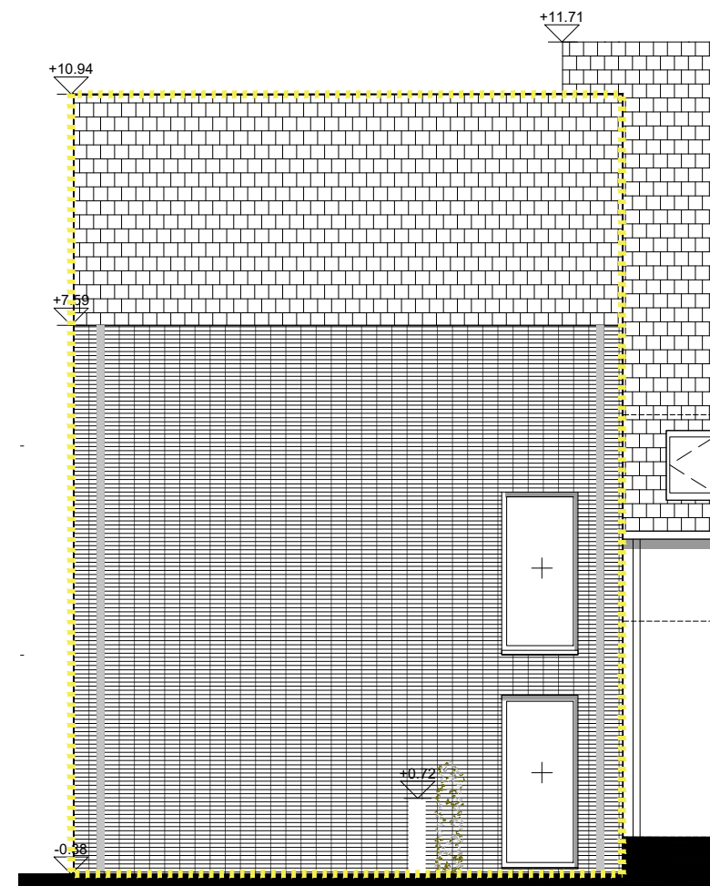
WEST GEVEL
