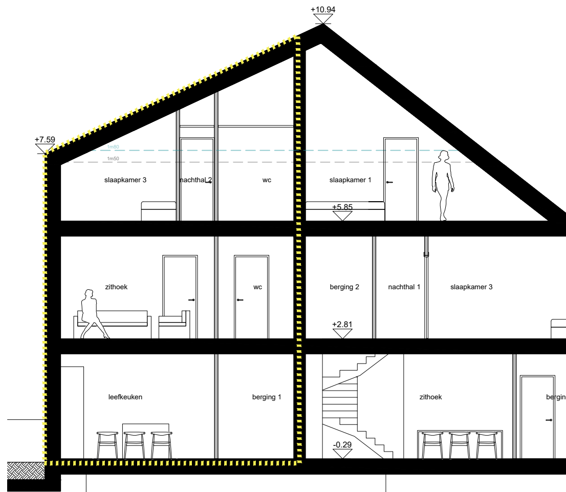
SNEDE E2
