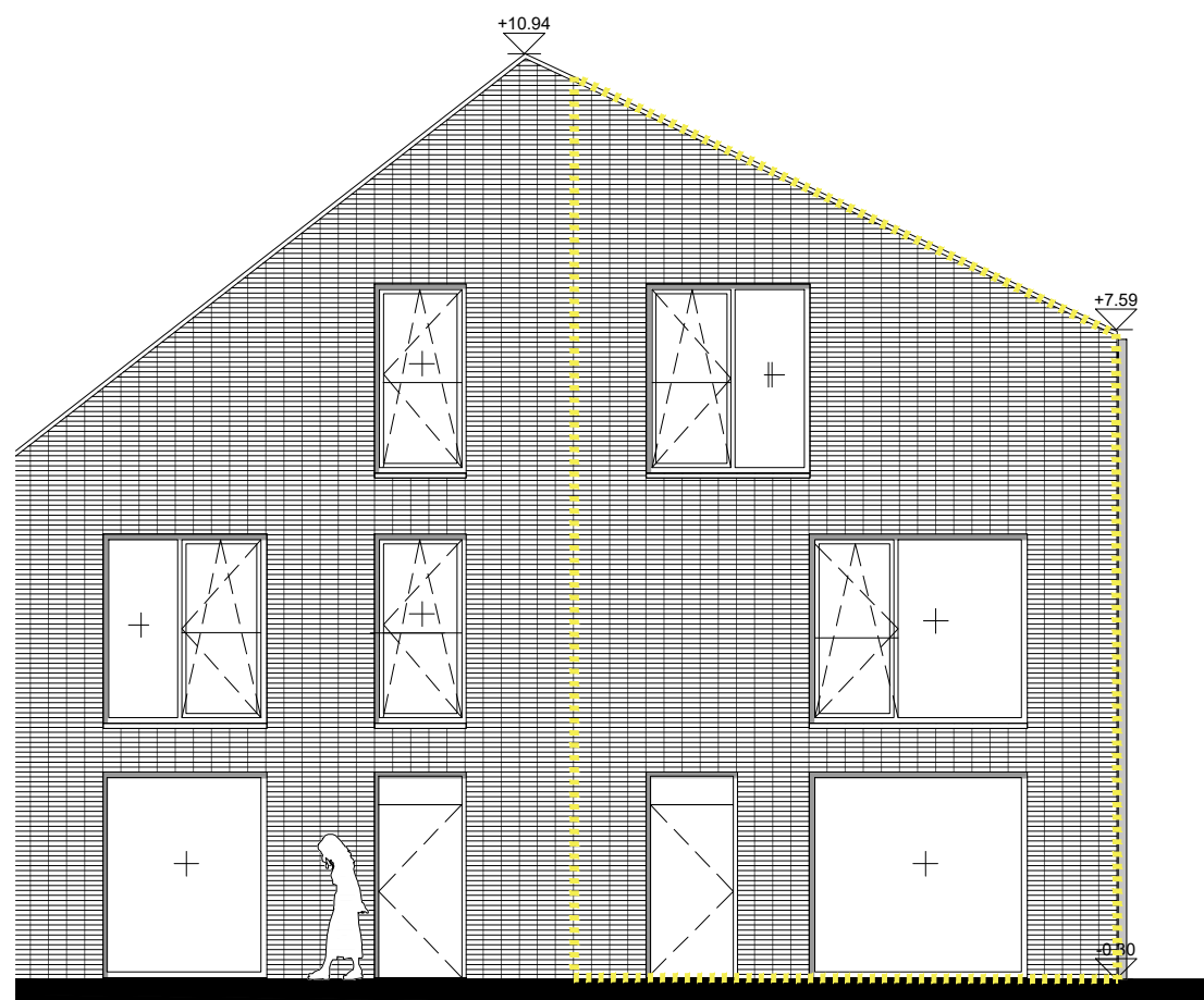
NOORD GEVEL
