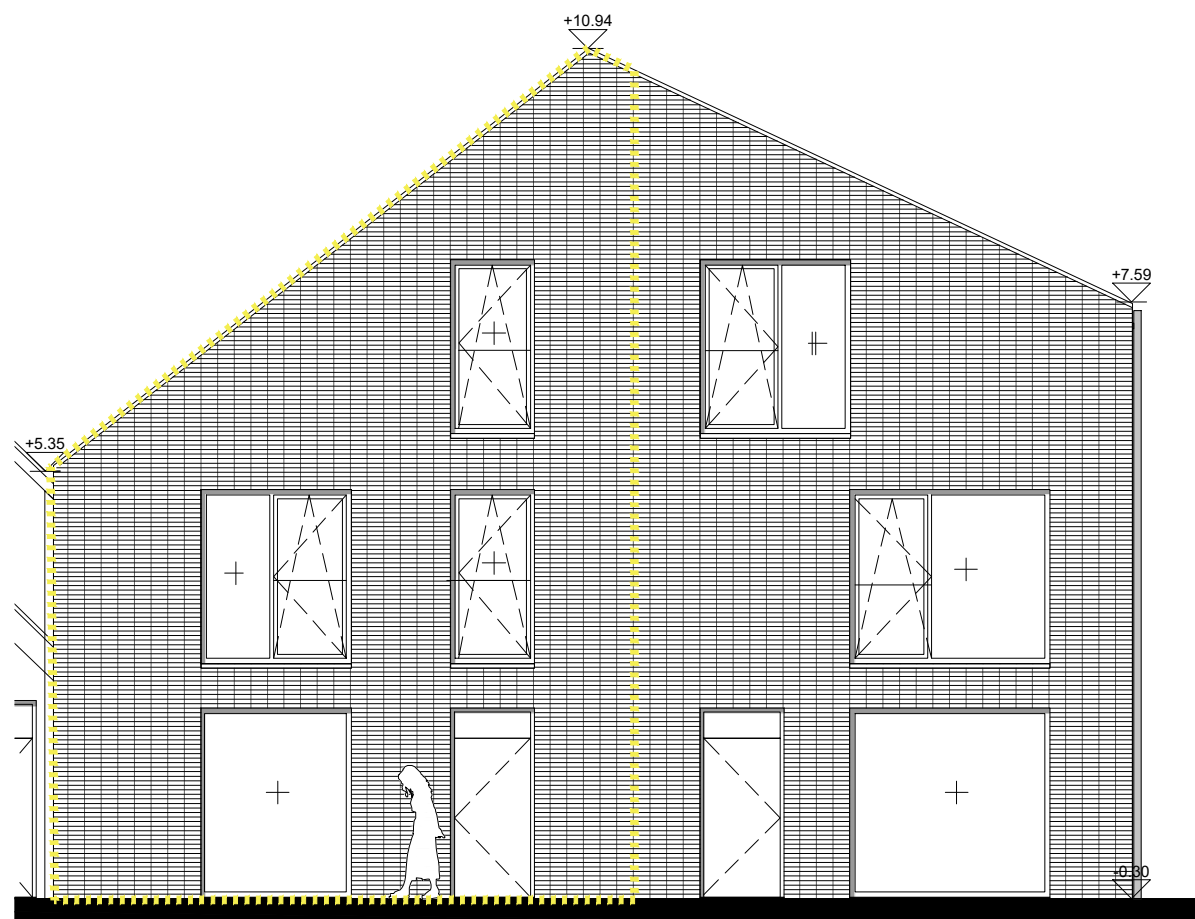
NOORD GEVEL
