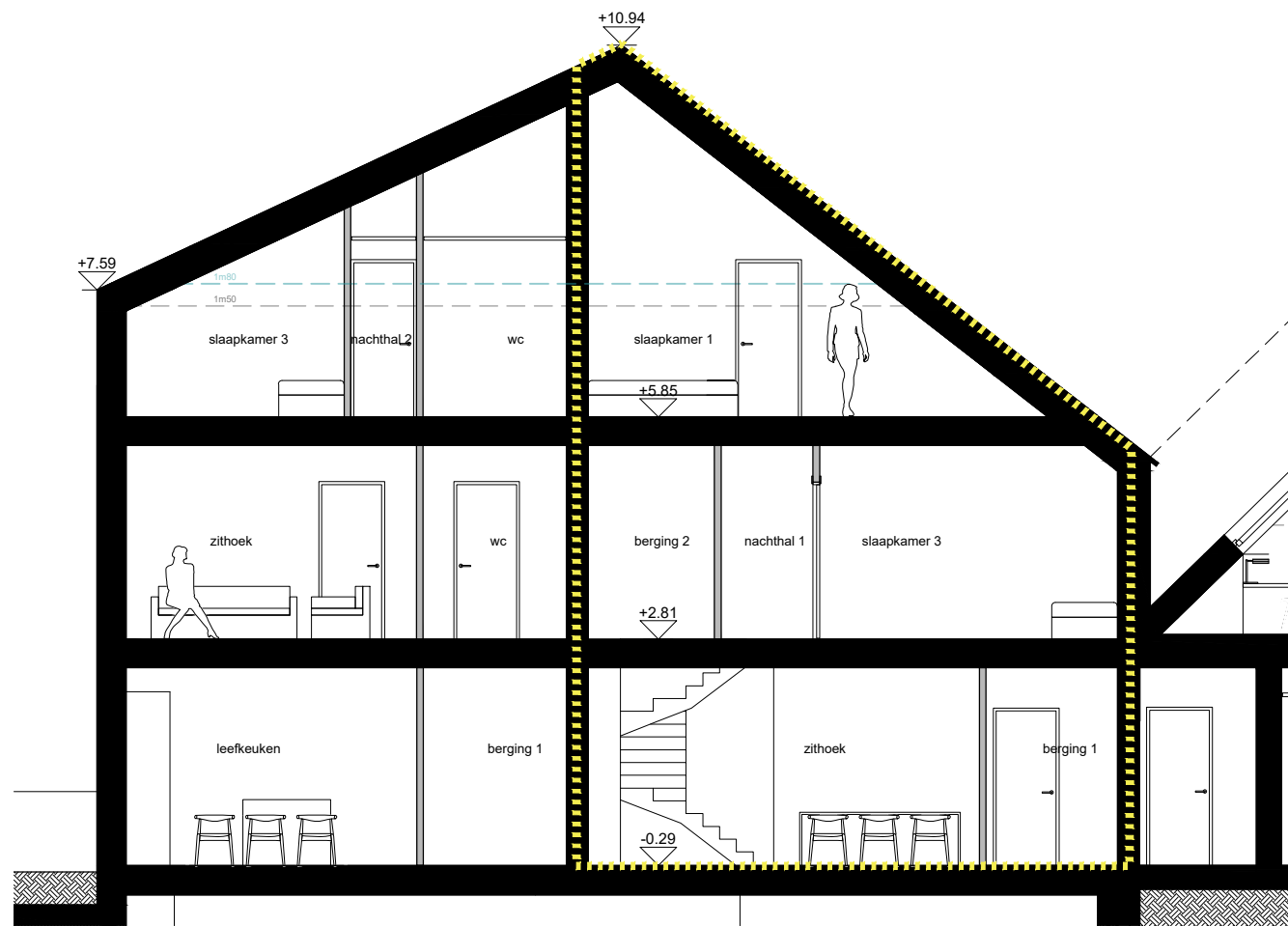
SNEDE E1
