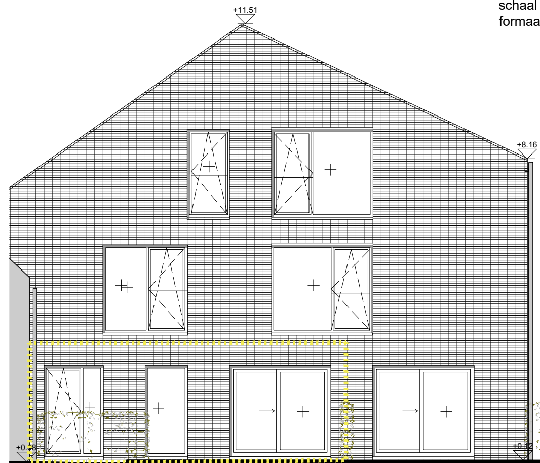
NOORD GEVEL
