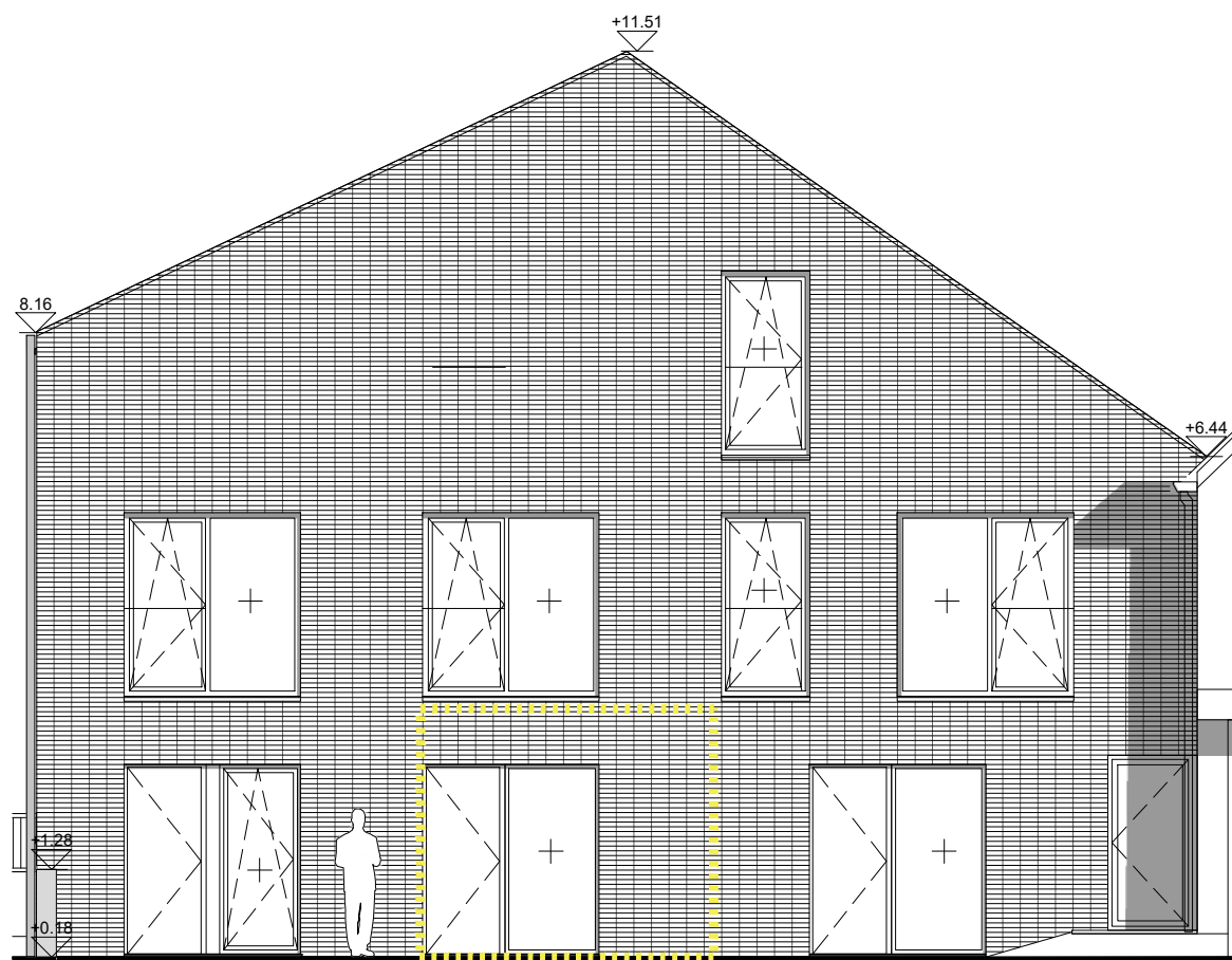
ZUID GEVEL
