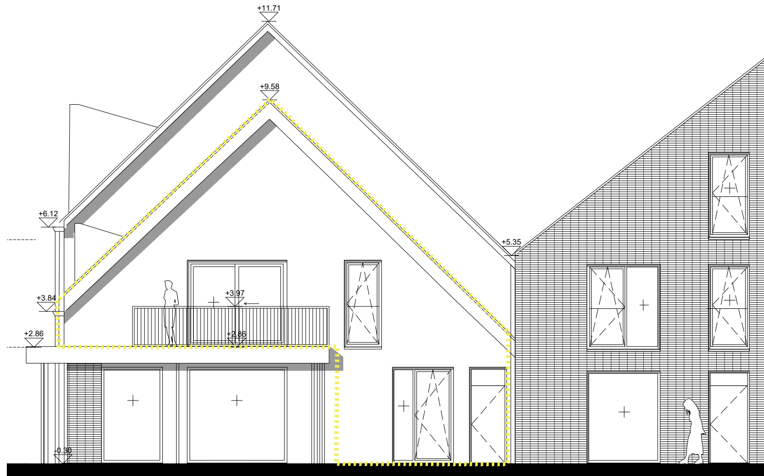
NOORD GEVEL
