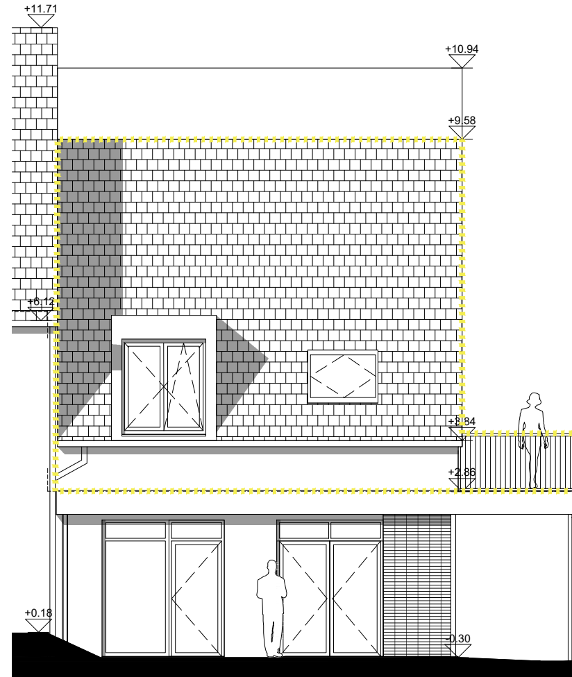
OOST GEVEL
