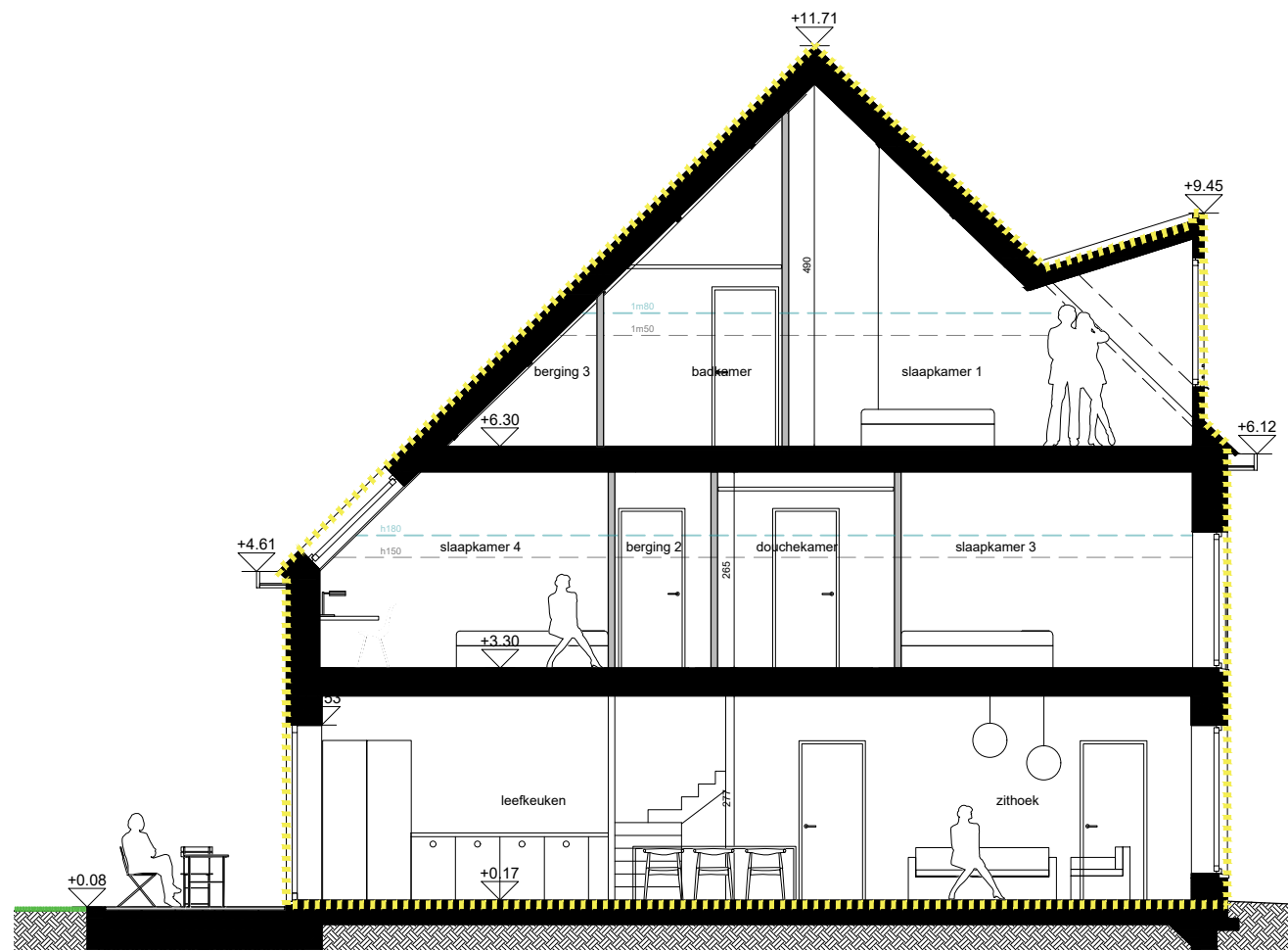
SNEDE C5
