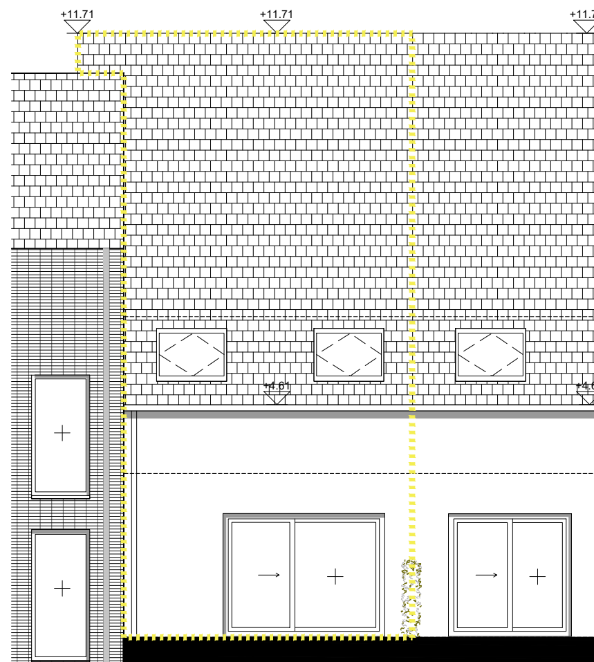
WEST GEVEL
