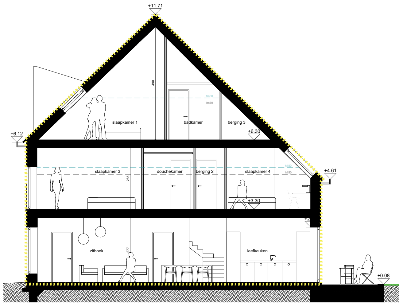
SNEDE C3
