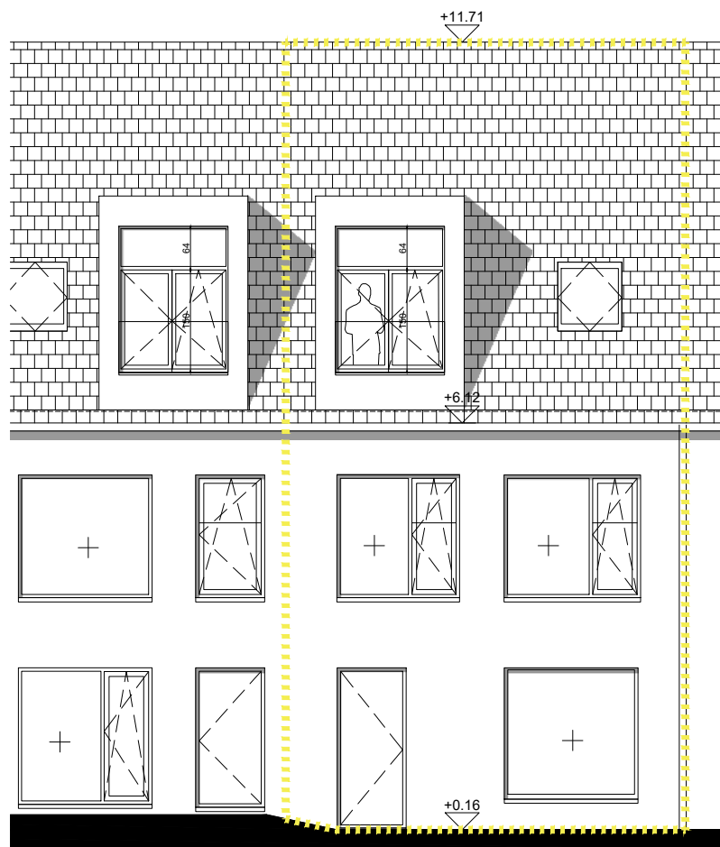
OOST GEVEL
