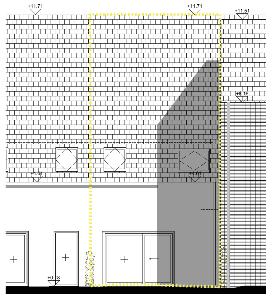
WEST GEVEL
