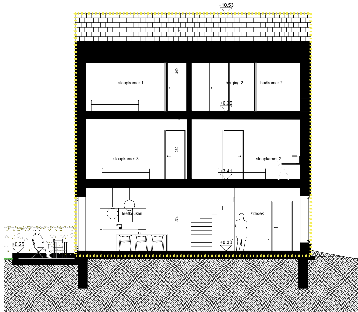
SNEDE A4
