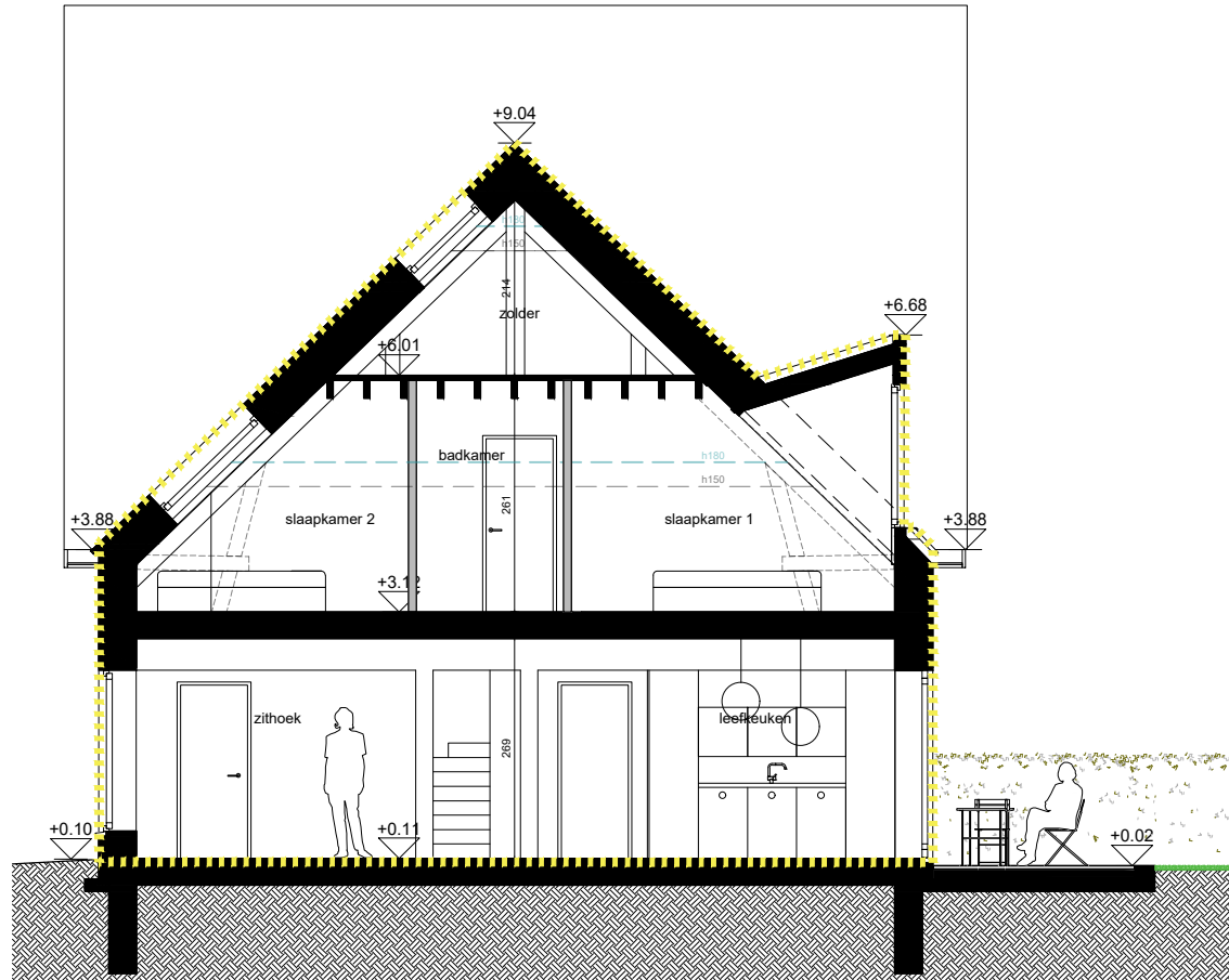
SNEDE A1
