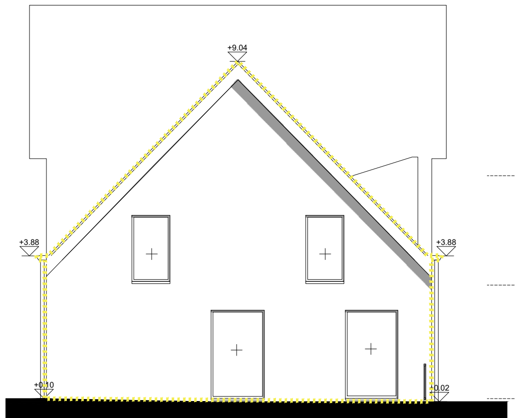
WEST GEVEL
